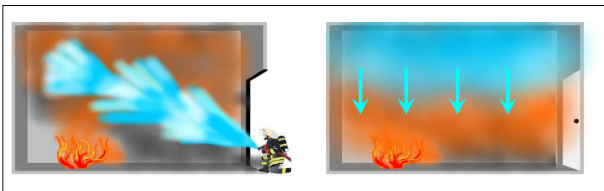
Abb. 10: Raumkühlung
